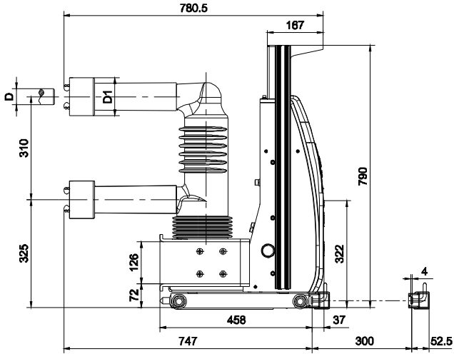
(4) 车轮处尺寸标注基准
