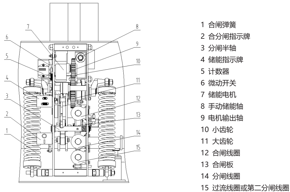
图 1 断路器操作机构正视
